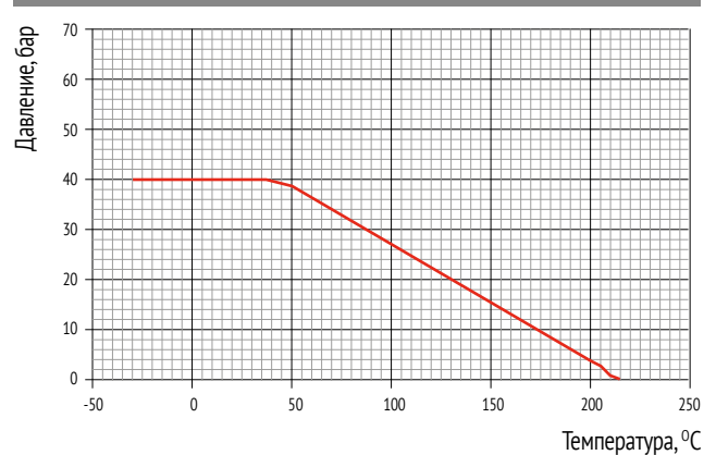
Диаграмма температура/давление
