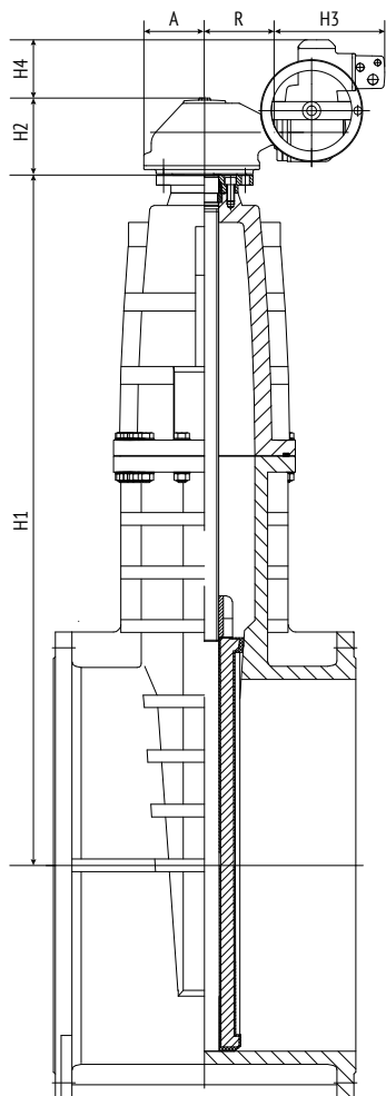
Технические характеристики DN700-1000
