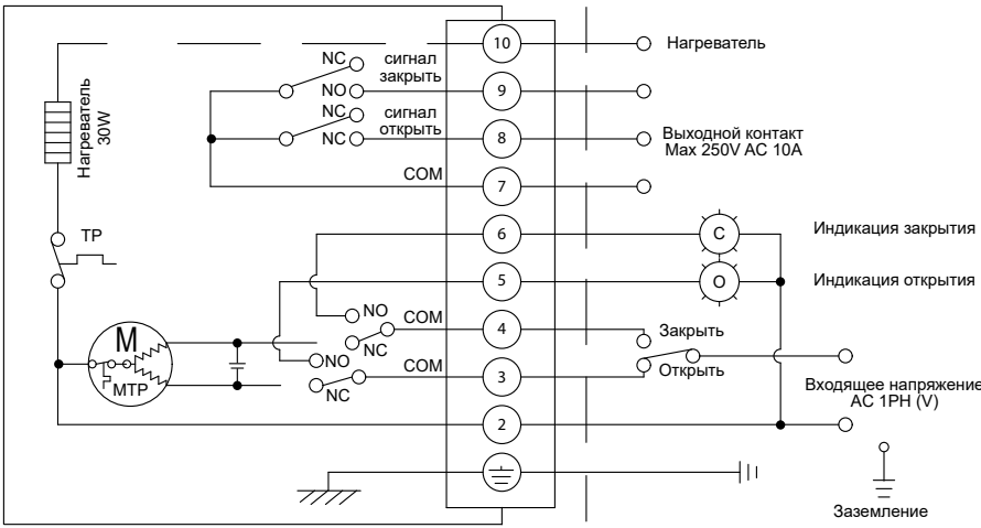
Схема подключения арт. 900, 220В
