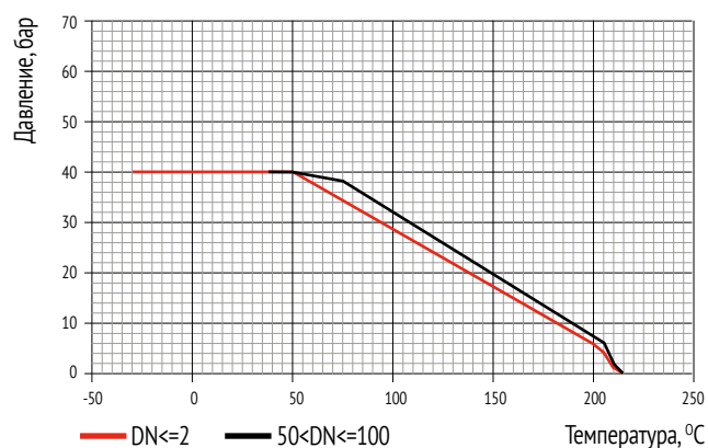
Диаграмма температура/давление
